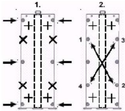
Рис. 8. Схема ослабления стяжных шпилек со стороны нажимной плиты
