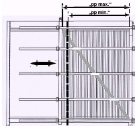
Рисунок 7. Размеры пакета пластин.
