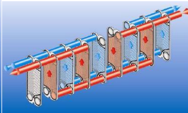
Рисунок 2. Многоходовая схема
