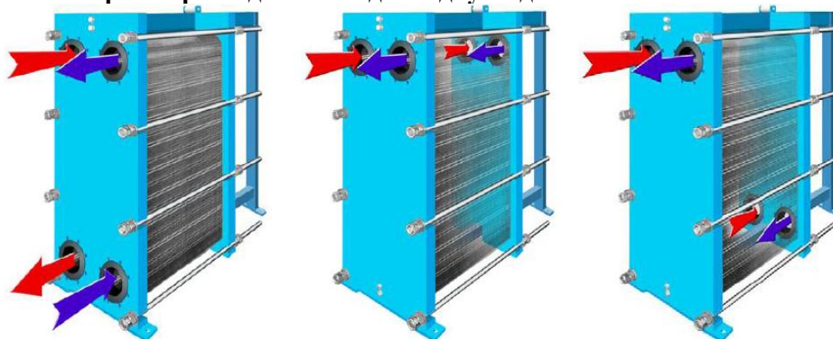
Одноходовая схема Двухходовая схема Трехходовая схема
