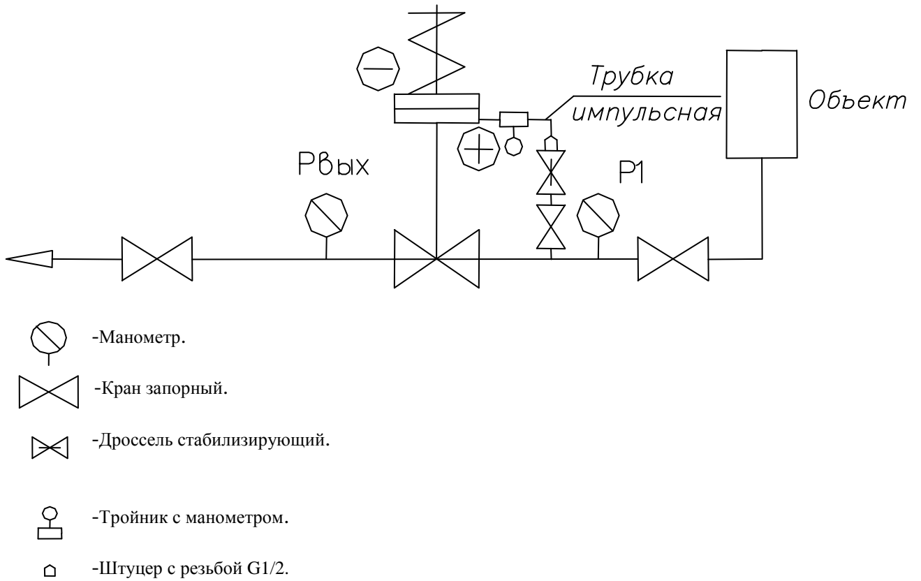
Рисунок 1. Схема подключения регулятора давления «до себя».
