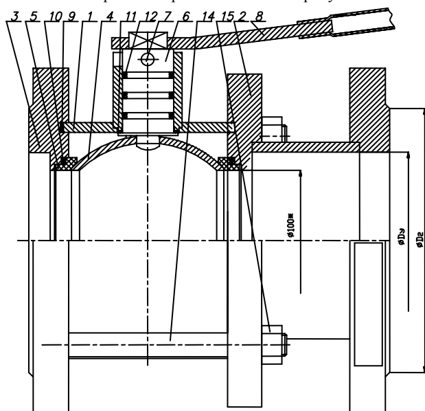
Рисунок 1. Общее устройство
